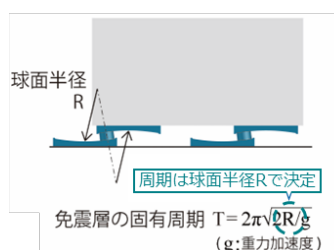
図1 積層ゴム免震とSSBの固有周期
